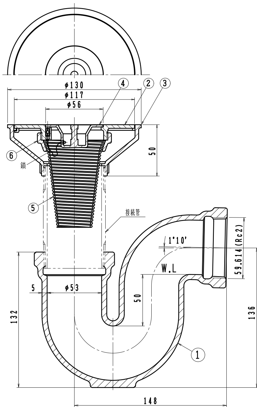
構成部品表
